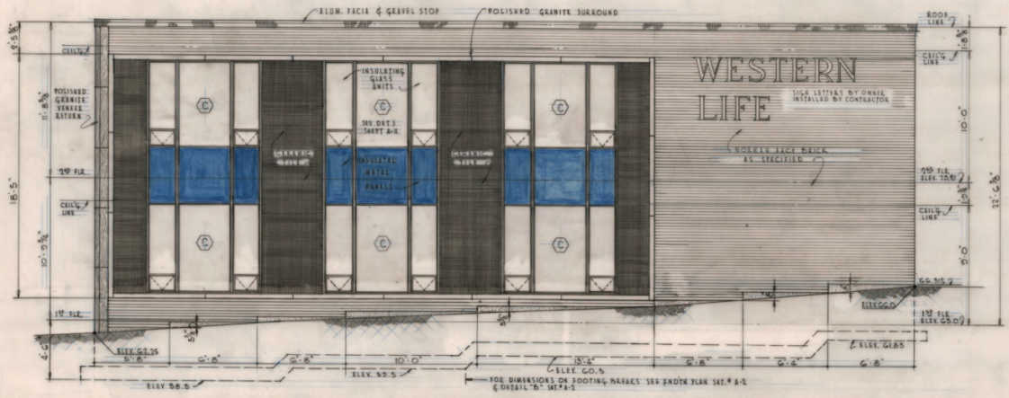
• NORTH ELEVATION • SCALE: 1/8" = 1'-0"
