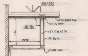
SOFFIT - DETAIL SCALE: 3/8" = 1'-0"
